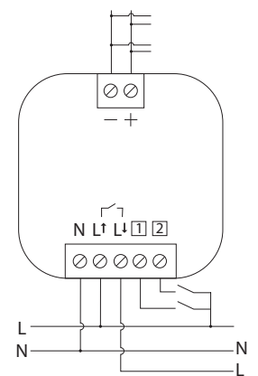
Kobling for 1-10 V buss (med avbrudd av forsyning til last)
