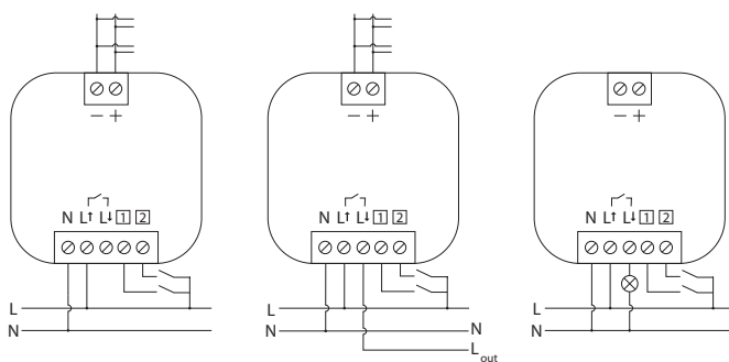
Aansluiting voor 0-10 V bus (zonder onderbreking van stroomtoevoer naar last)
