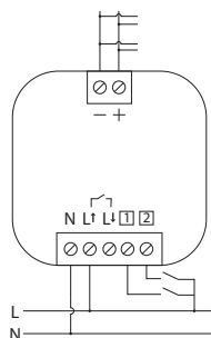
Koppling för 0-10 V bus (utan brytning av matning till last)
