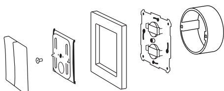
Montage utanpå apparatdosor med skruv.
